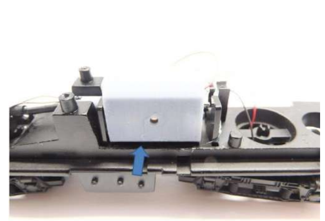
Motor kleben Glue the motor Lijm de motor
