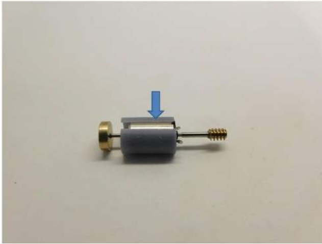
Der Motor wird mit Epoxidkleber oder Sekundenkleber in den Motorhalterteile eingeklebt The motor is glued into the motor holder parts with epoxy glue or super glue De motor wordt verlijmd met secondelijm of epoxy lijm
