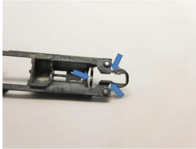
Schaffen Sie Platz für das Schnecke Make extra room for the worm gear Maak ruimte voor het wormwiel
