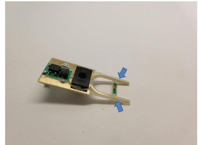
Platine kürzen Shorten PCB Kort de printplaat in
