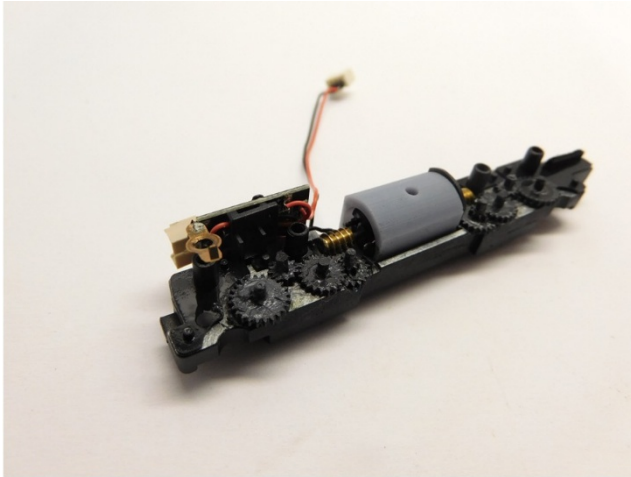
Löten Sie die Drähte Solder the wires Soldeer de draden Rot, Red - / Schwarz, black +
