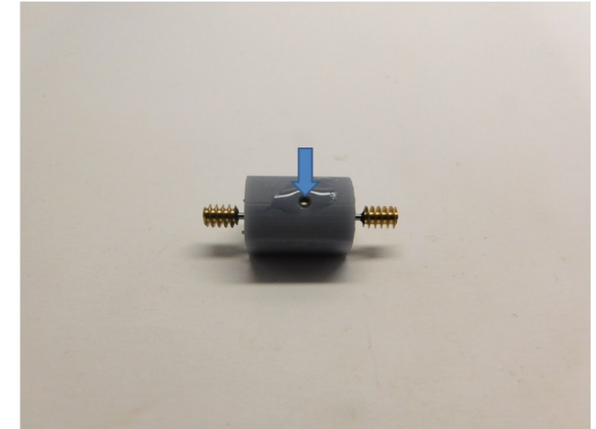
Der Motor wird mit Sekundenkleber in den Motorhalterteile eingeklebt The motor is glued into the motor holder parts with super glue De motor wordt verlijmd met secondelijm of epoxy lijm
