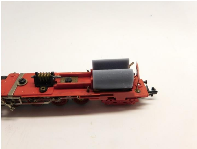
Platzieren Sie den Motorhalter Place the motor holder Plaats de motorhouder
