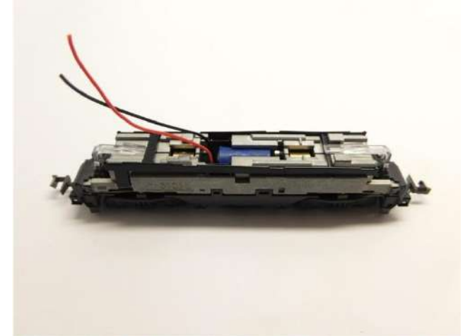
Drehgestelle platzieren Place the bogies Plaats de draaistellen
