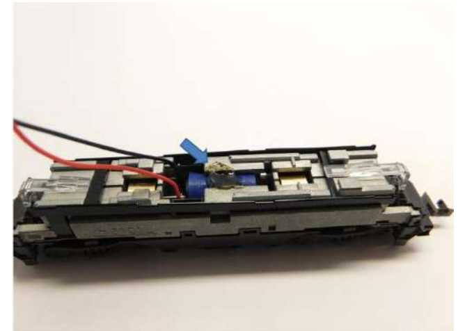
Motor kleben (Heizkleber) Glue the motor (Hotmelt) Lijm de motor (lijmpistool)
