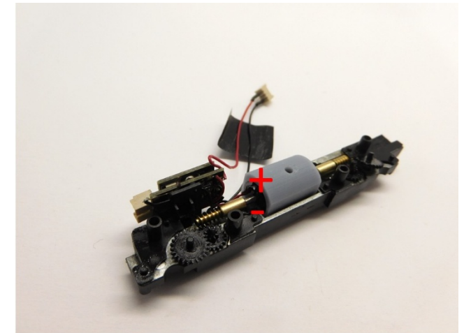
Löten Sie die Drähte Solder the wires Soldeer de draden Rot, Red - / Schwarz, black +
