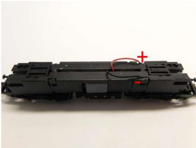
Drähte am Rahmen befestigen Clamp wires to frame Klem de draden aan het frame
