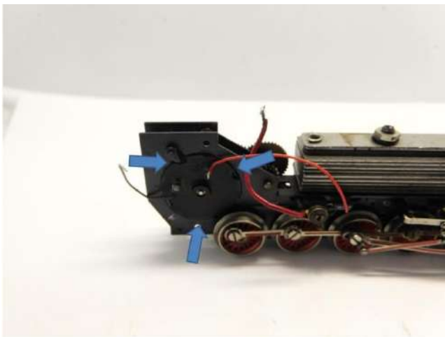
Motor kleber Glue motor Verlijm de motor
