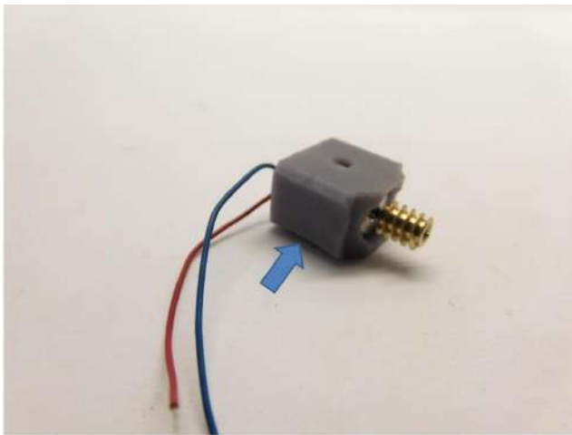
Die Ecken schräg feilen File the corners at an angle Vijl de hoeken schuin af
