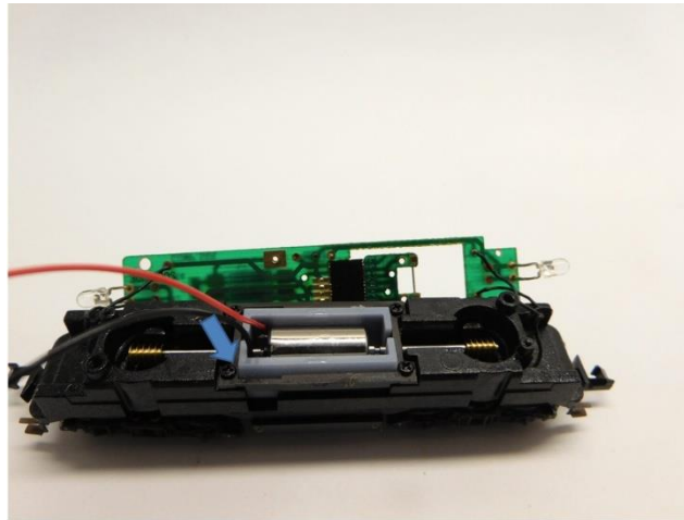
Rahmen platzieren Mount frame
