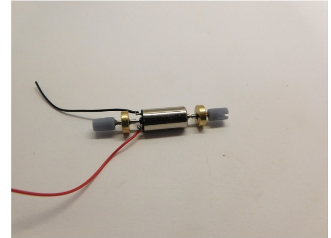
Kleben die Kardankupplungshalter Glue the cardan coupler shafts Verlijm de kardankoppelingshouders
