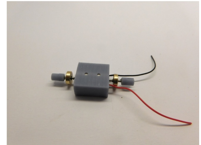
Platzieren Sie den Motor in die Halter Place the motor in the holder Plaats de motor in de motor houder
