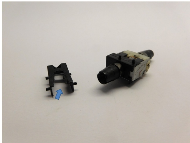
Sie brauchen diese Teile wieder. Diese werden mit einem scharfen Messer entfernt You need the parts again. They can be removed with sharp knife Je hebt deze onderdelen wederom nodig. Ze kunnen met een scherp mes verwijderd worden
