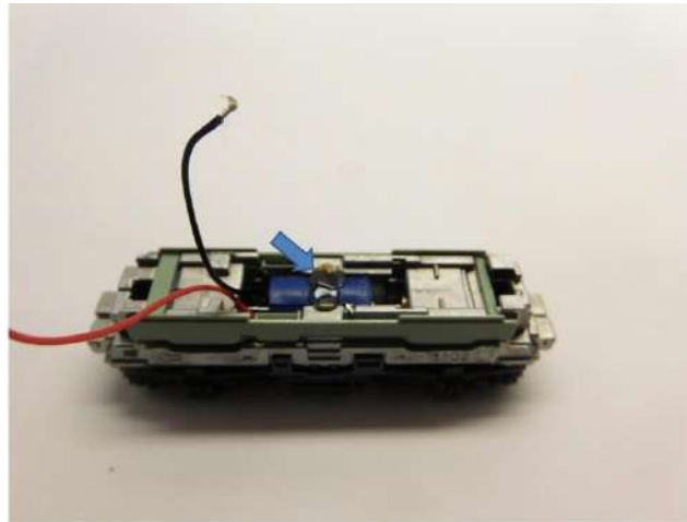
Motor kleben (Heizkleber) Glue the motor (Hotmelt) Lijm de motor (Lijmpistool)
